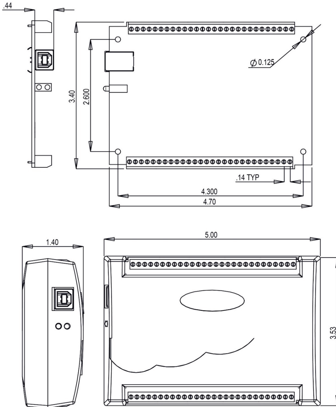
Abbildung 11. Leiterplatte des RedLab 1808X (oben) und Gehäusemaße
