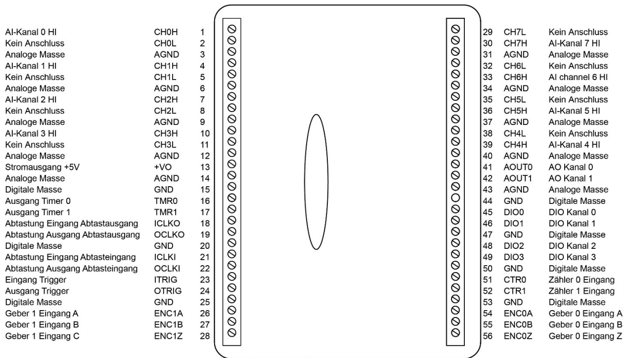
Abbildung 3. SE-Pinbelegung
