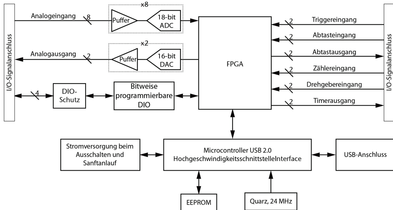
Abbildung 1. Funktionsdiagramm
